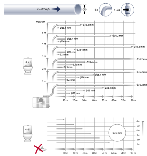
Sololift2 WC-1
