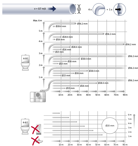
Sololift2 WC-3
